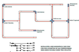
ESQUEMA DE CONEXIONES EN LOS CARRILES TRIFÁSICOS
